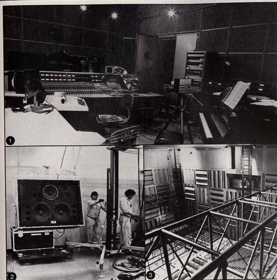
1. Studio III de l'I.R.C.A.M. 2. Une enceinte des studios de l'I.R.C.A.M. (Photo Teycheney). 3. Recherche et essai sur l'acoustique : panneaux amovibles (Photo J.P. Armand)
