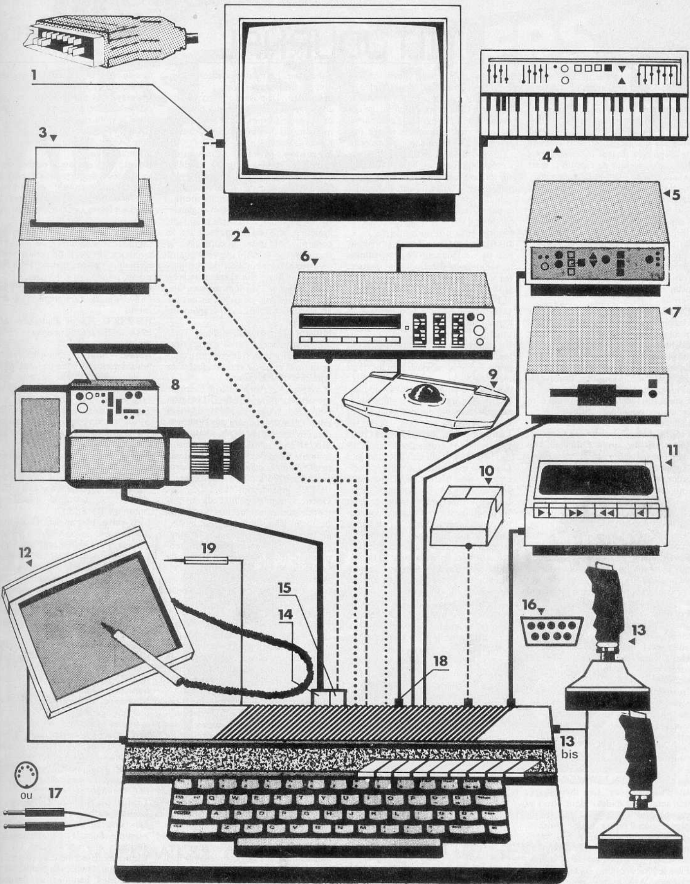
1 - Prise Pritel 2 - Moniteur 3 - Imprimante 4 - Synthétiseur 5 - Modem 6 - Lecteur de disques numériques 7 - Lecteur de disquettes 8 - Caméra vidéo 9 - Trackball 10 - Souris 11 - Lecteur de cassettes 12 - Tablette graphique 13 - Manettes de jeu 13 bis - Interface manettes de jeu 14 - Extension incrustation/digitalisation 15 - Interface Pritel 16 - Prise pour manette de jeu 17 - Prise pour raccord magnétophone 18 - Prise MIDI 19 - Stylo optique.
